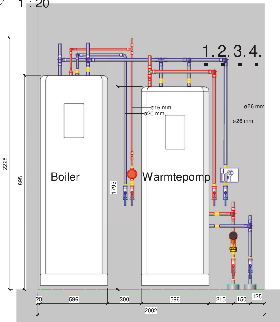
Vooraanzicht Calibra Duo
